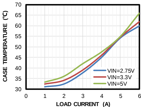
Thermal Rise
