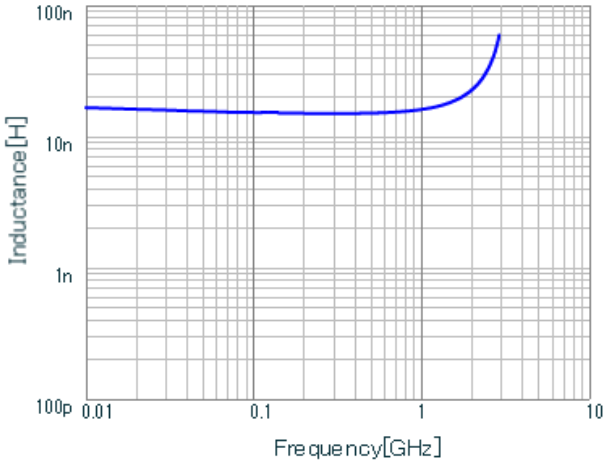
LQG15WZ15NG02 L.
